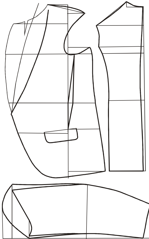
Рис. 1. Чертеж конструкции мужского смокинга конца XIX века
