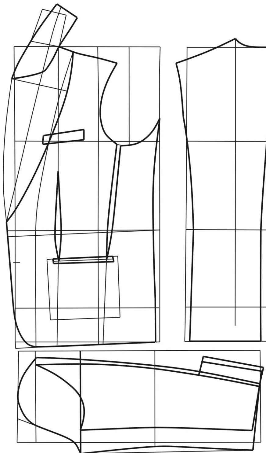
Рис. 2. Чертеж конструкции мужского смокинга начала XXI века
