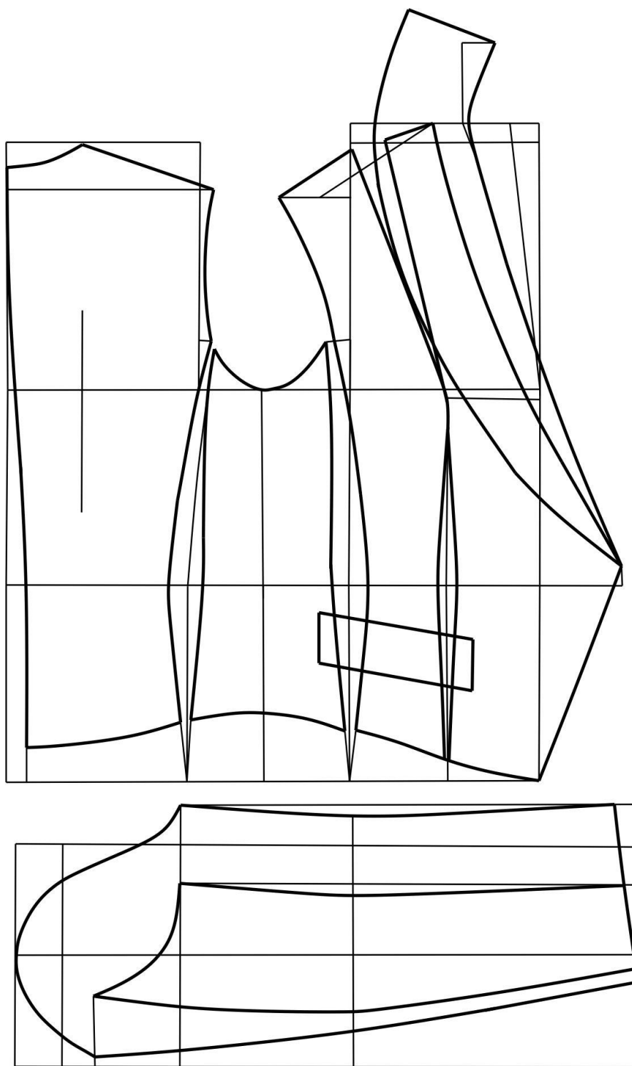
Рис. 3. Чертеж конструкции женского смокинга начала XXI века
