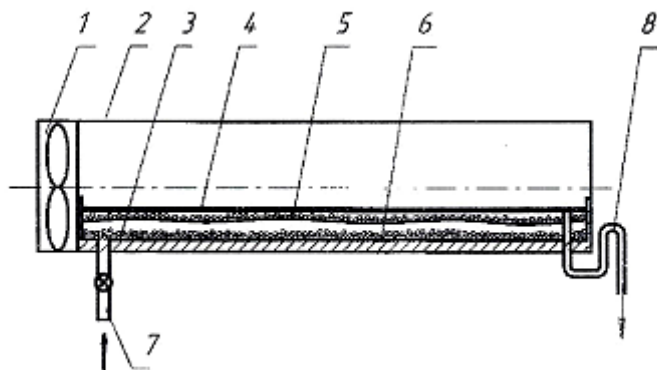
Рис. 1. Схема устройства для комбинированной сорбционной очистки и обеззараживания воздуха
