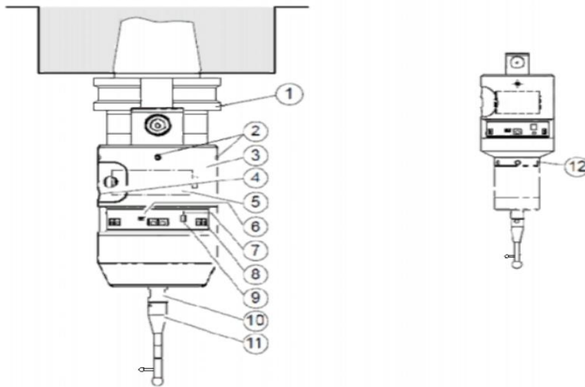
Рис. 1. Описание измерительного щупа BLUM TC51-20 1 – державка инструмента Komet ABS; 2 – центрирующие винты; 3 – отсек для батареи; 4 – обозначение прибора; 5 – батарея; 6 – Датчик Холла; 7 – светодиоды состояния (расположение под 120^\circ = 3 шт.) 8 – диоды передатчика (расположение под 60^\circ = 12 шт.); 9 – диоды приемника (расположение под 120^\circ = 3 шт.); 10 – измерительный механизм;
